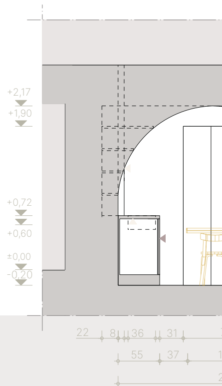
schnitt y-y cucina | küche
