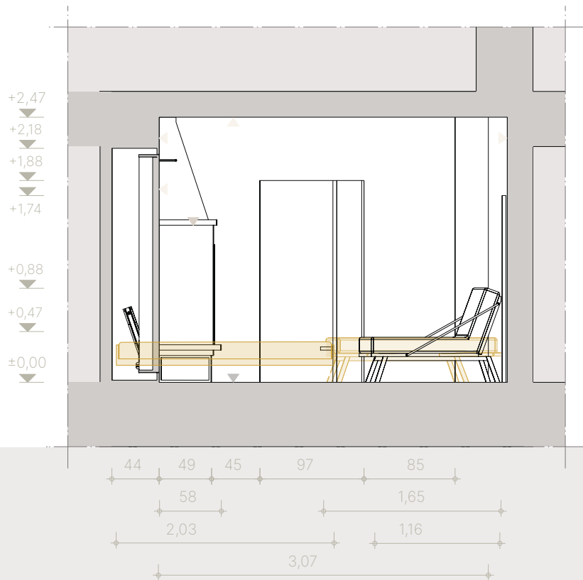
schnitt x-x zona giorno-notte | wohn-schlafbereich
