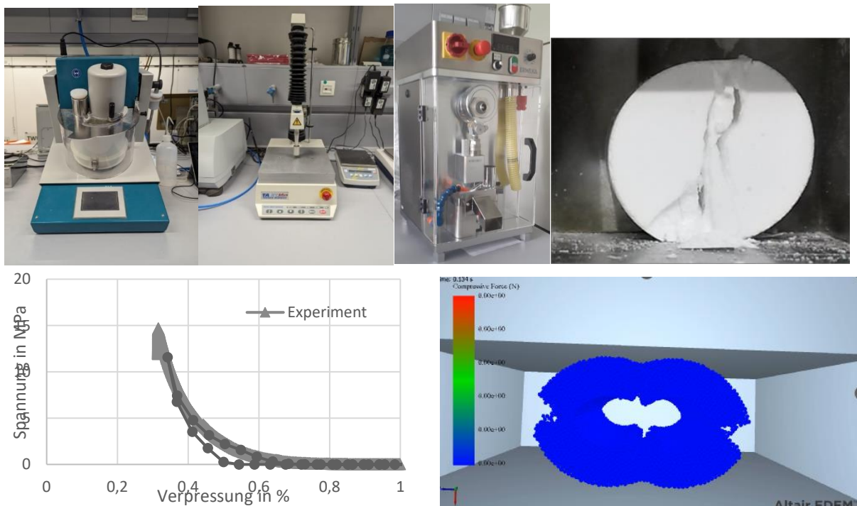
Abbildung 1: Intensivmischer; Texture Analyzer; Tablettenpresse; gebrochene Tablette; ermittelte Kraft-Weg-Kurve in Simulation und Experiment; Bruch eines Hohlkörpers über Simulation in der Diskreten Elemente Methode
