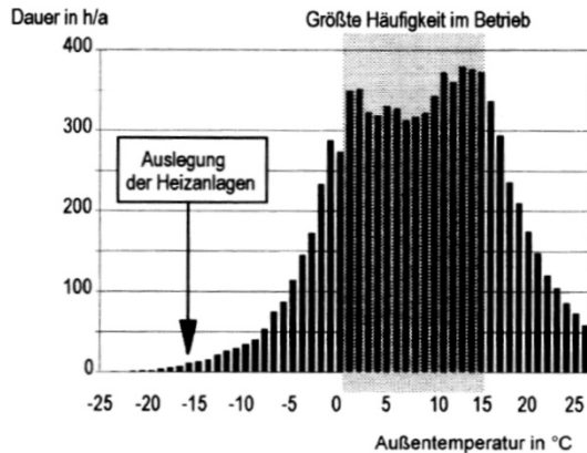
Stunden pro Jahr nach Außentemperatur – München
