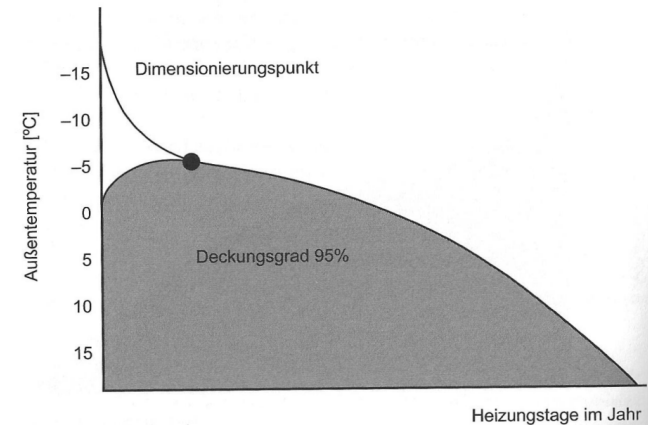
Bivalent – ca. 95 % durch Wärmepumpe, Rest Heizstab
