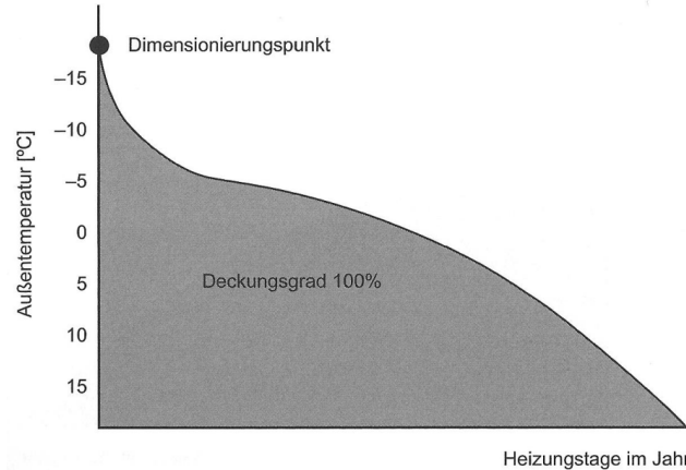
Monovalent 100 % durch Wärmepumpe
